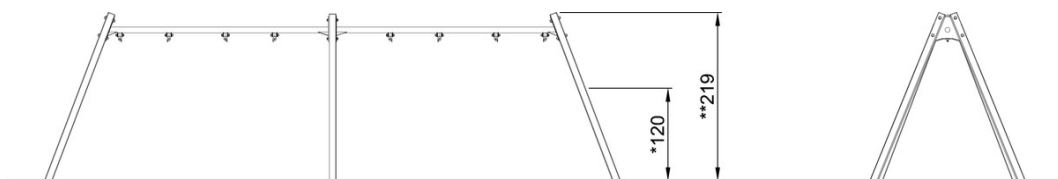
KPL902-xx01 1:300
